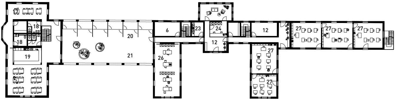
gelijkvloers
