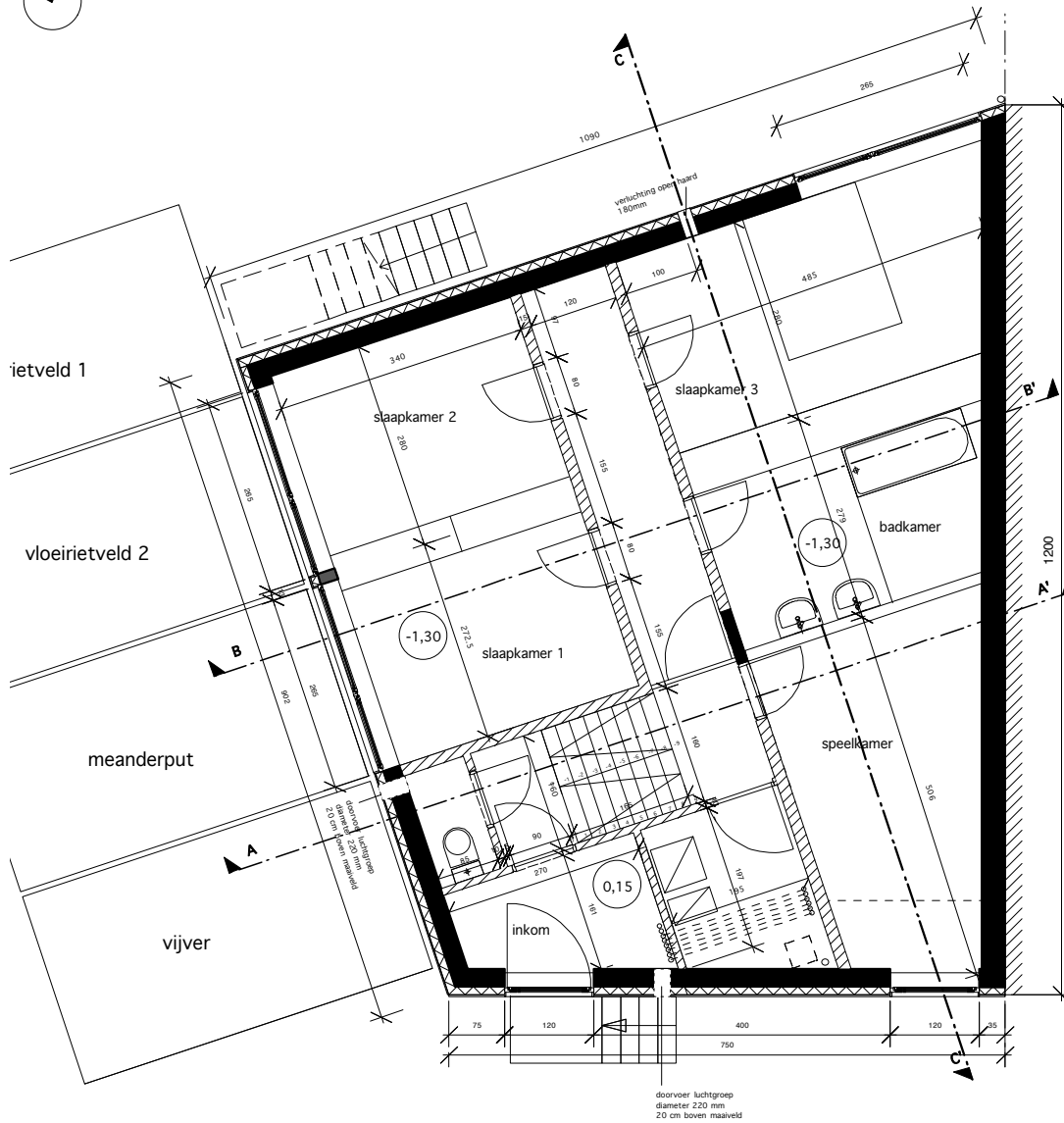
woning Dekeyzer 02 SOUS-SOL schaal 1/100
