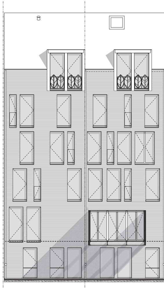
ACHTERGEVEL
