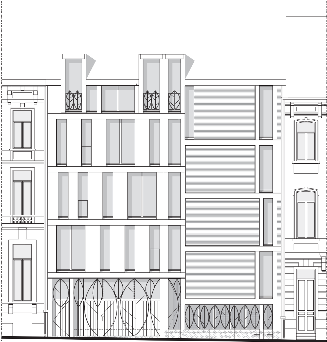
VOORGEVEL
