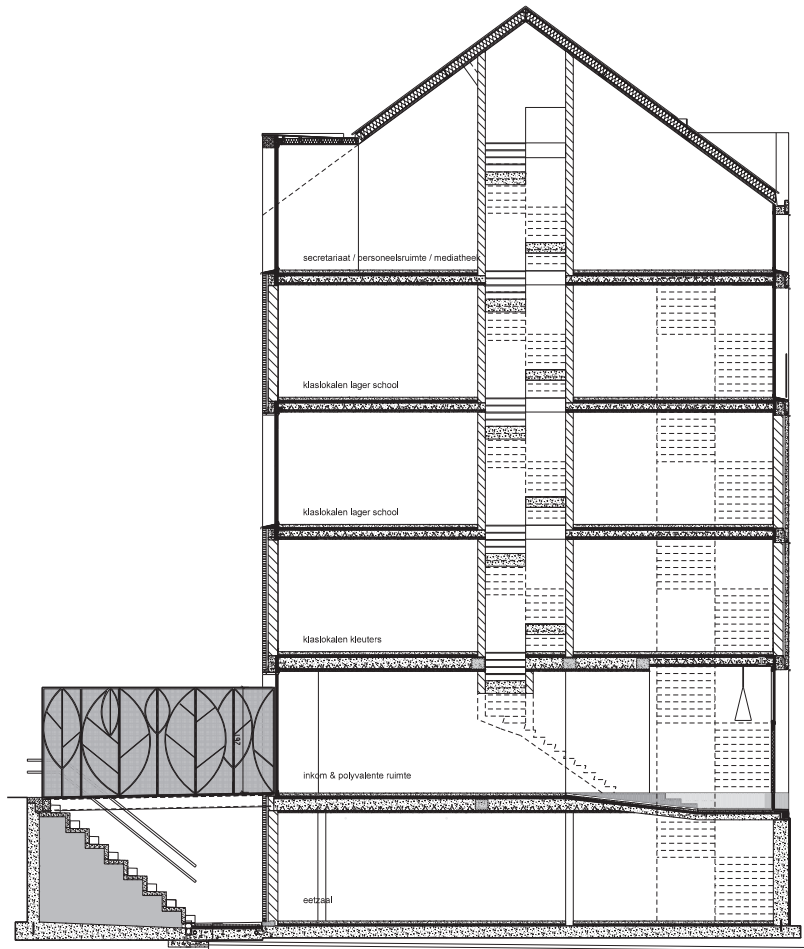
DOORSNEDE AA
