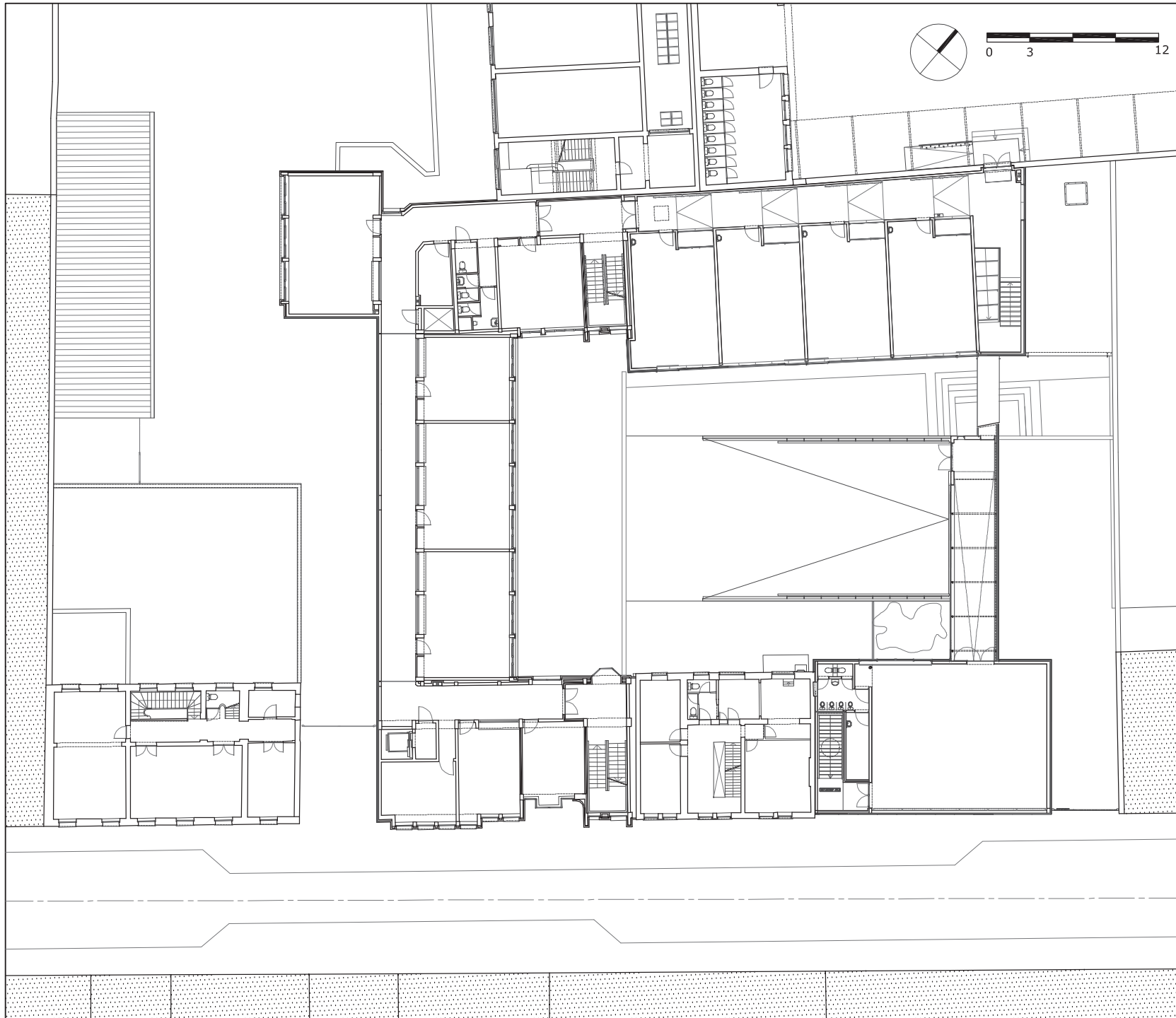
plan eerste verdieping
