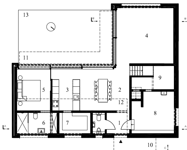
Gelijkvloers 1:200
