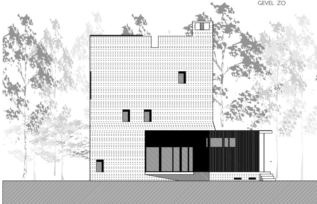
GEVEL NW
