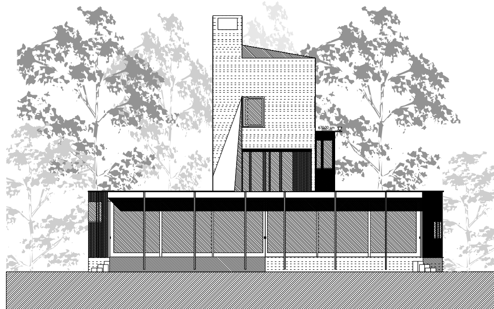
GEVEL ZW
