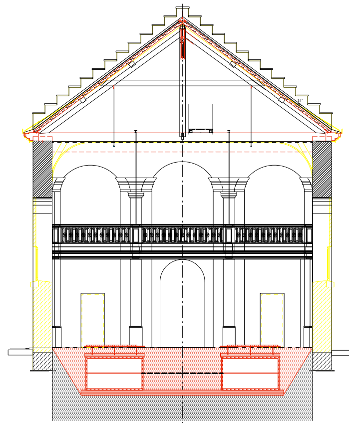
DOORSNEDE B GRAFKELDER
