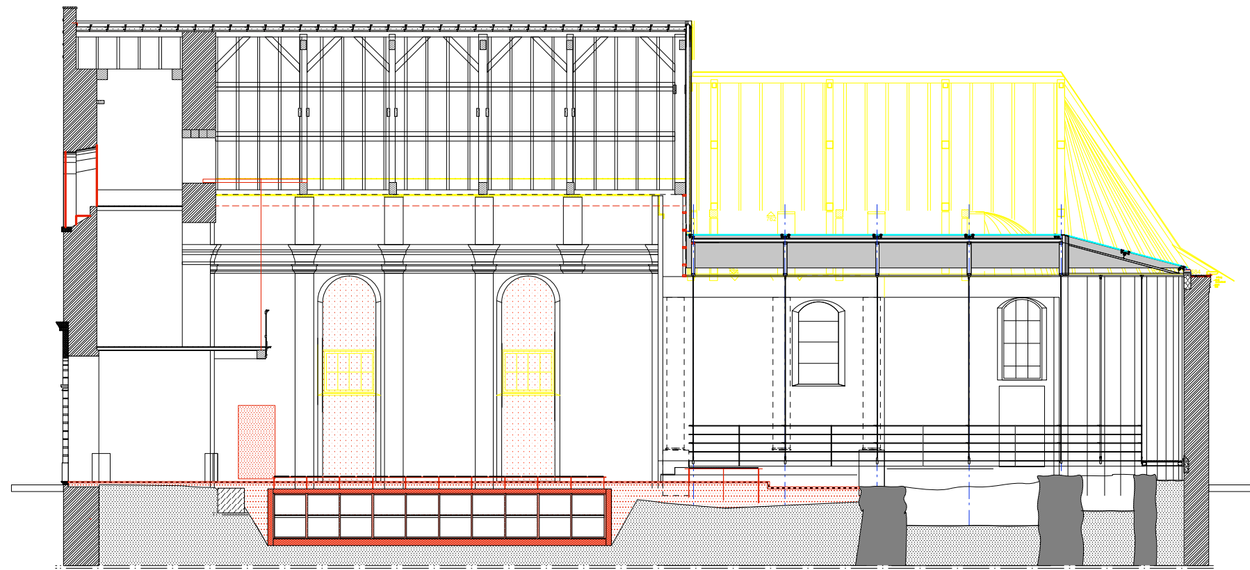
LANGSDOORSNEDE E GRAFKELDER
