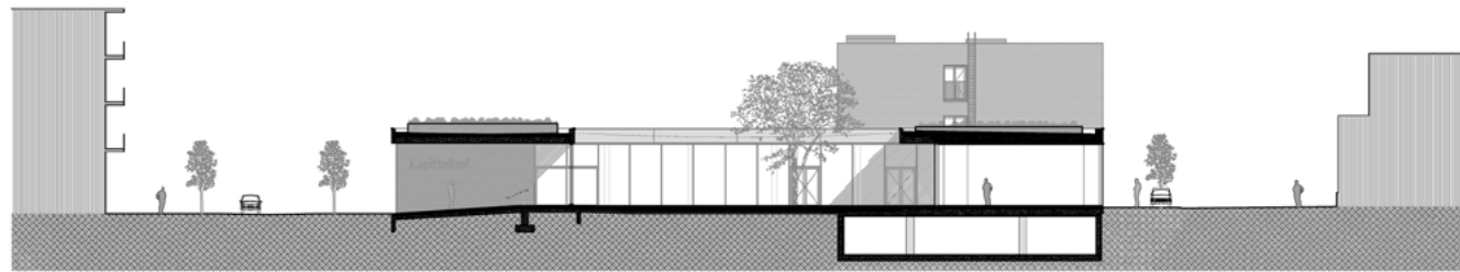
snede BB
