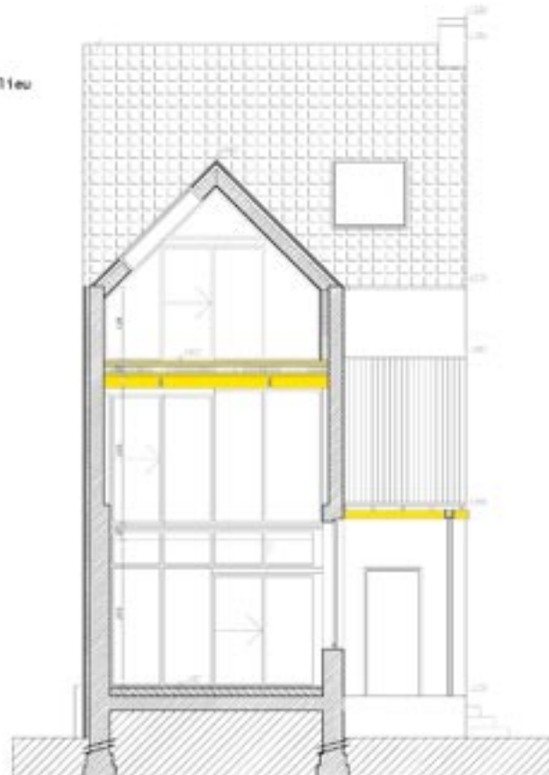
DOORSNEDE BB
