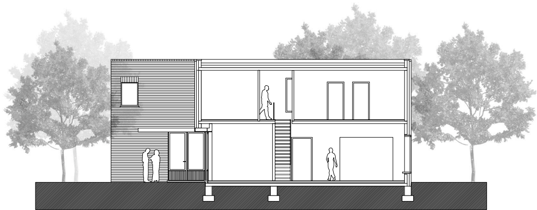
dwarse snede
