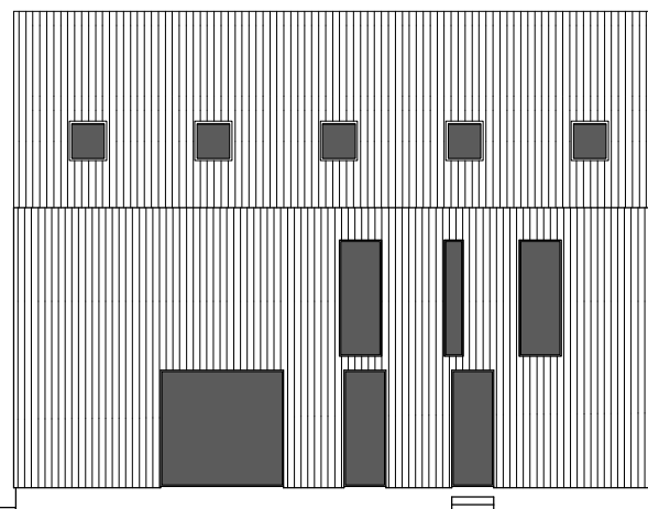
OOSTGEVEL
