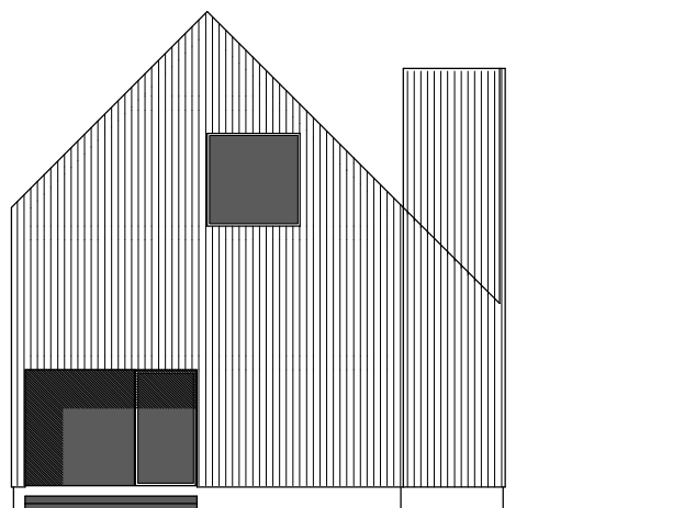
VOORGEVEL
