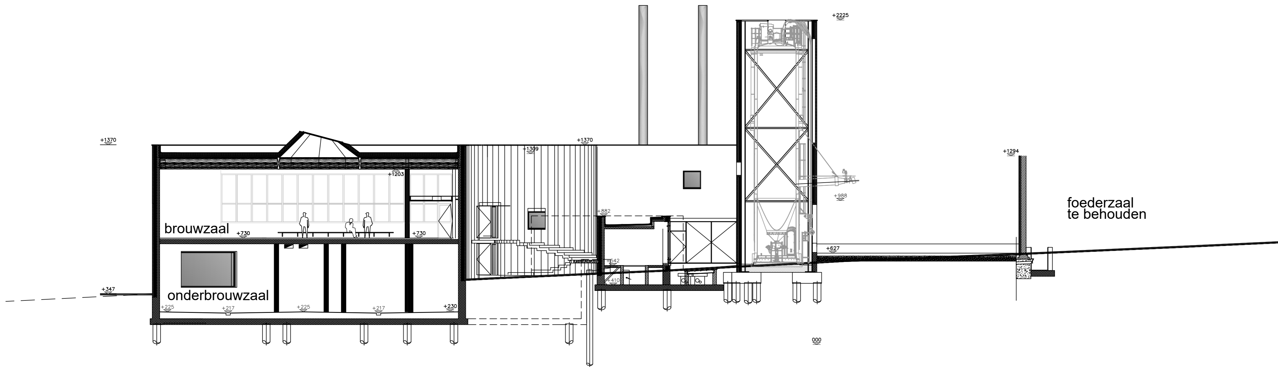
DOORSNEDE 1-1'
