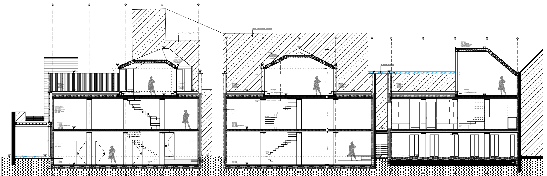
doorsnede over woningen en kantoor
