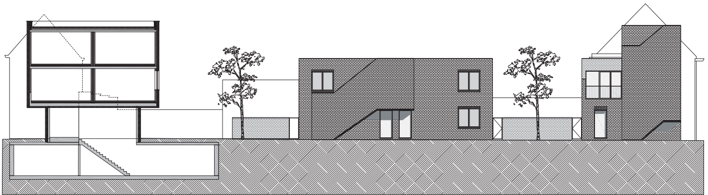
Binnenstraat Snede A-A'
