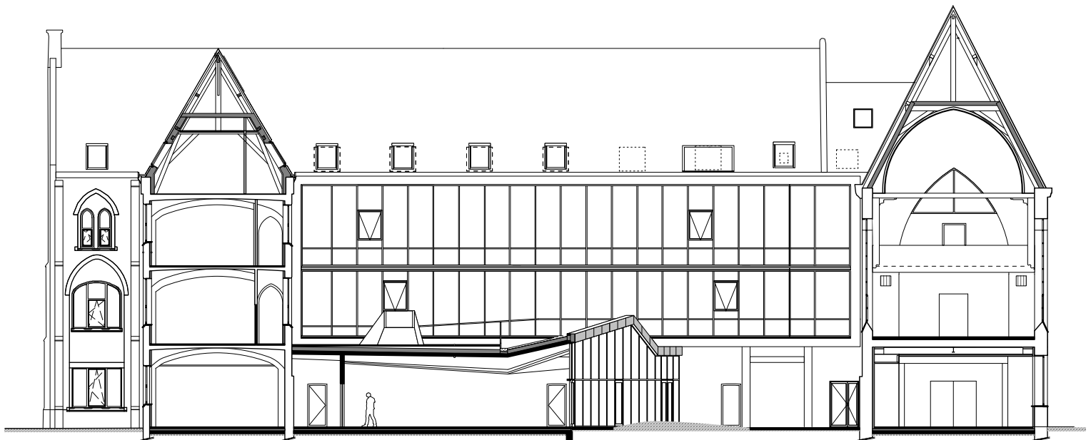
DOORSNEDES BB'
