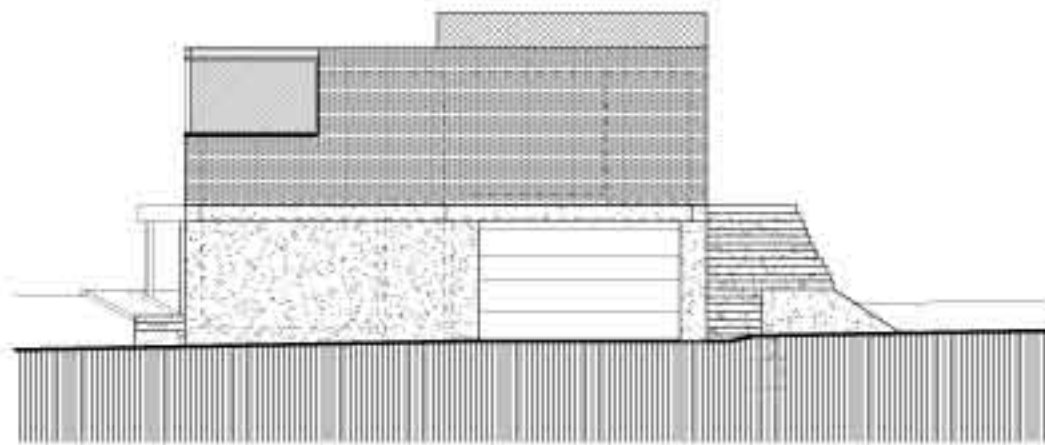
voorgevel
