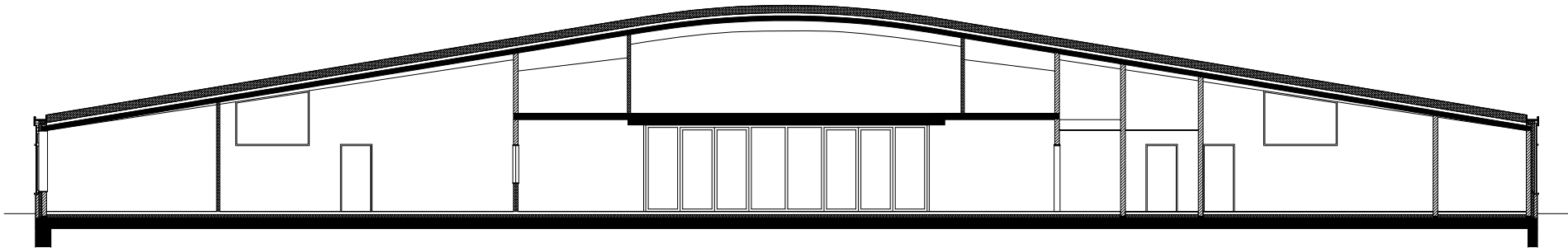
BB' 1/200
