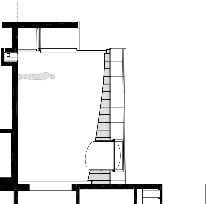
sneede A-A scale 1/100
