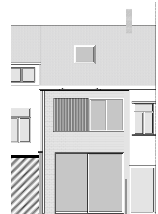
ACHTERGEVEL S 1/100
