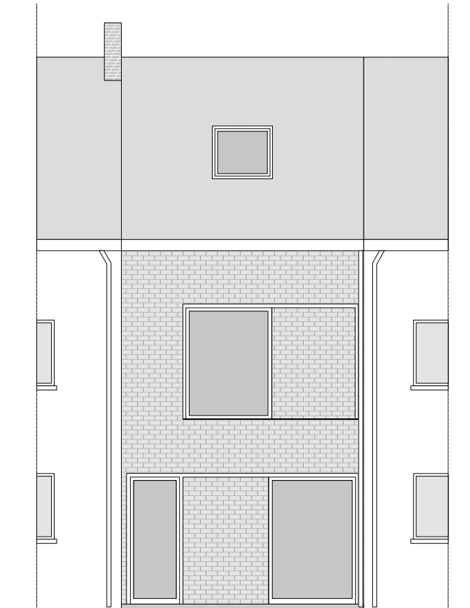
VOORGEVEL S 1/100
