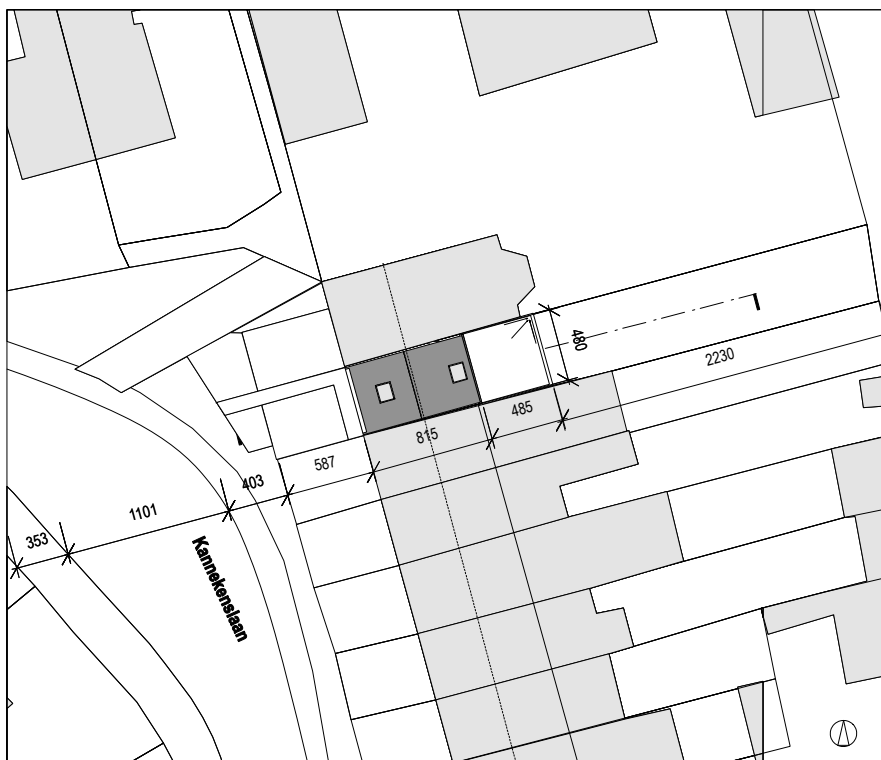
INPLANTINGSPLAN NIEUW S 1/500
