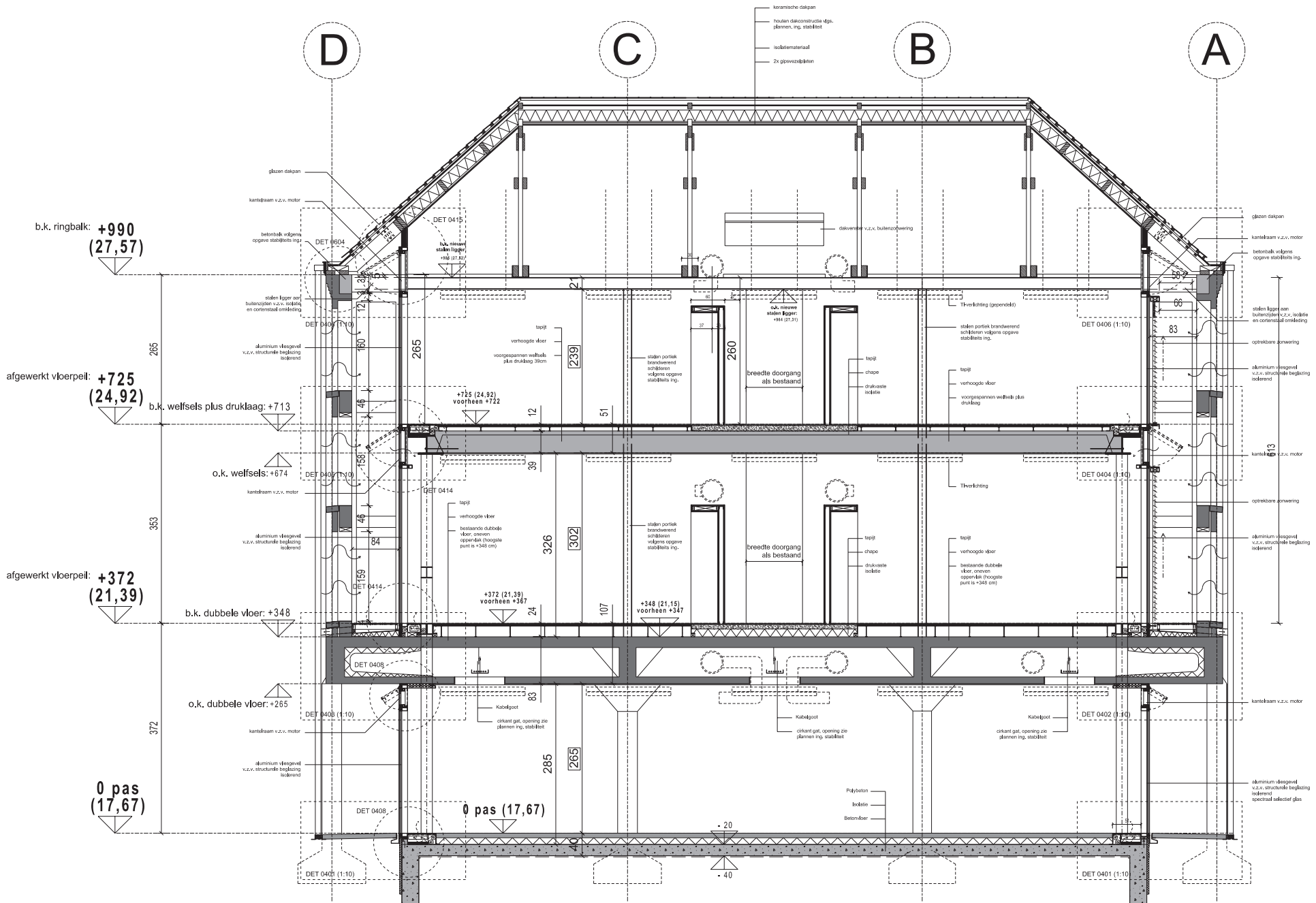
Doorsnede B-B (1:50)
