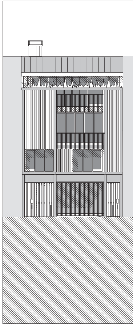
zuidgevel Ketelvest
