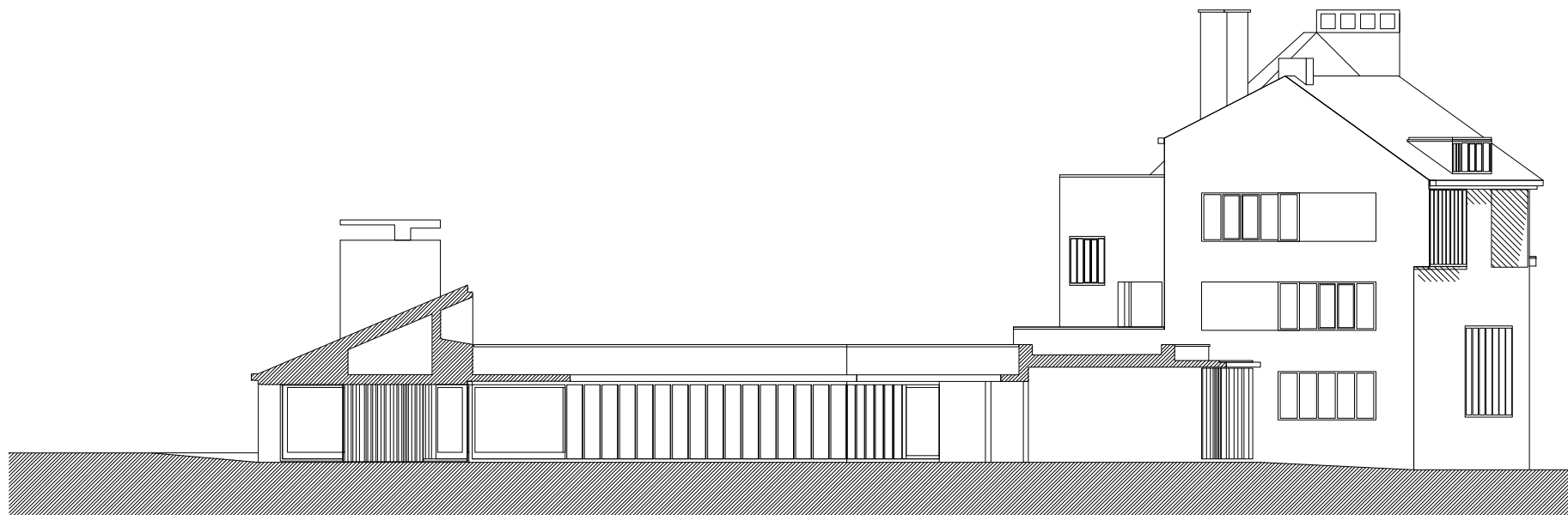
aanzicht west, zijgevel en gevel grote binnentuin
