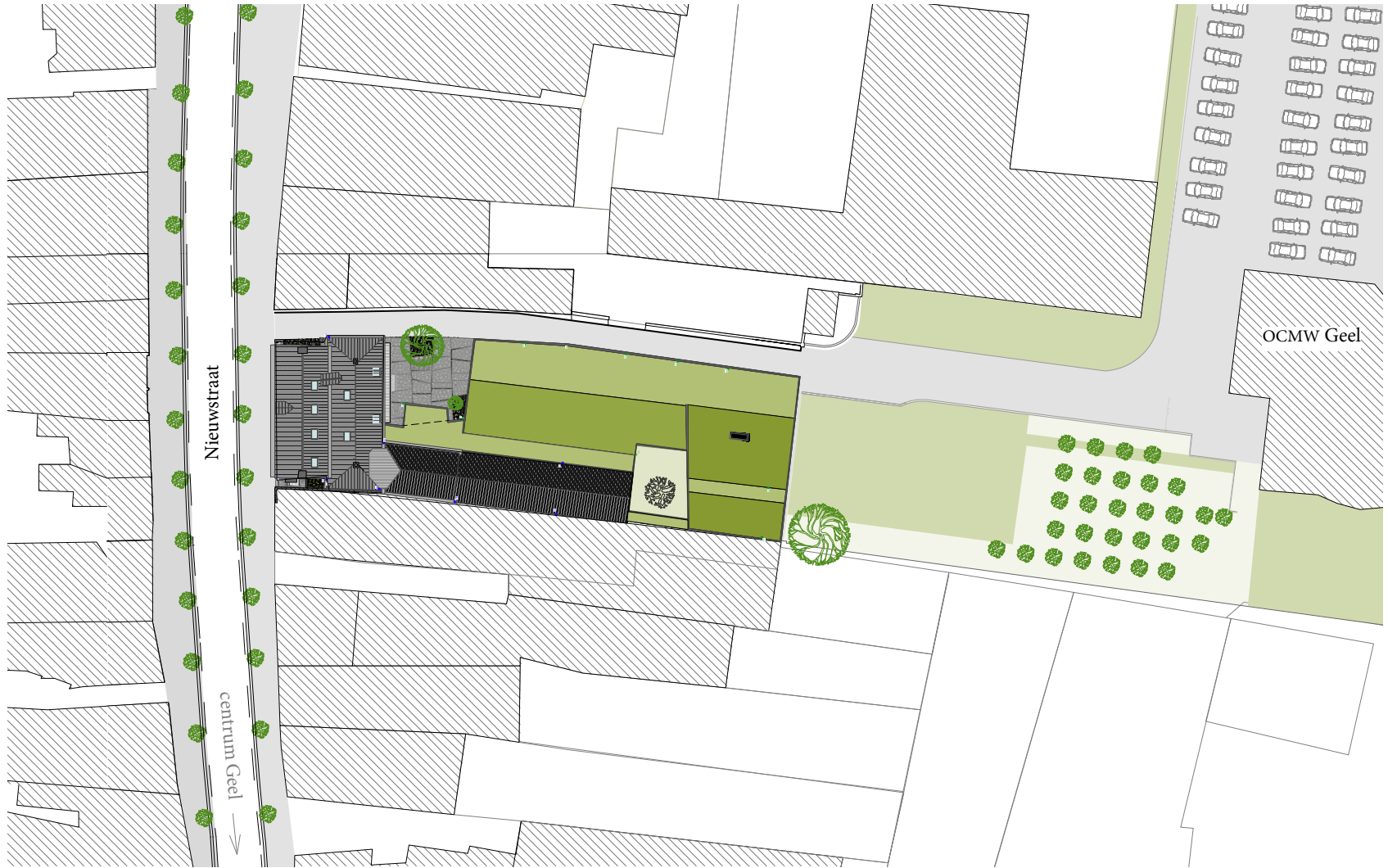
plan 1 inplantingsplan m u r m u r architecten i.s.m. Robbrecht en Daem architecten (adviseur)
