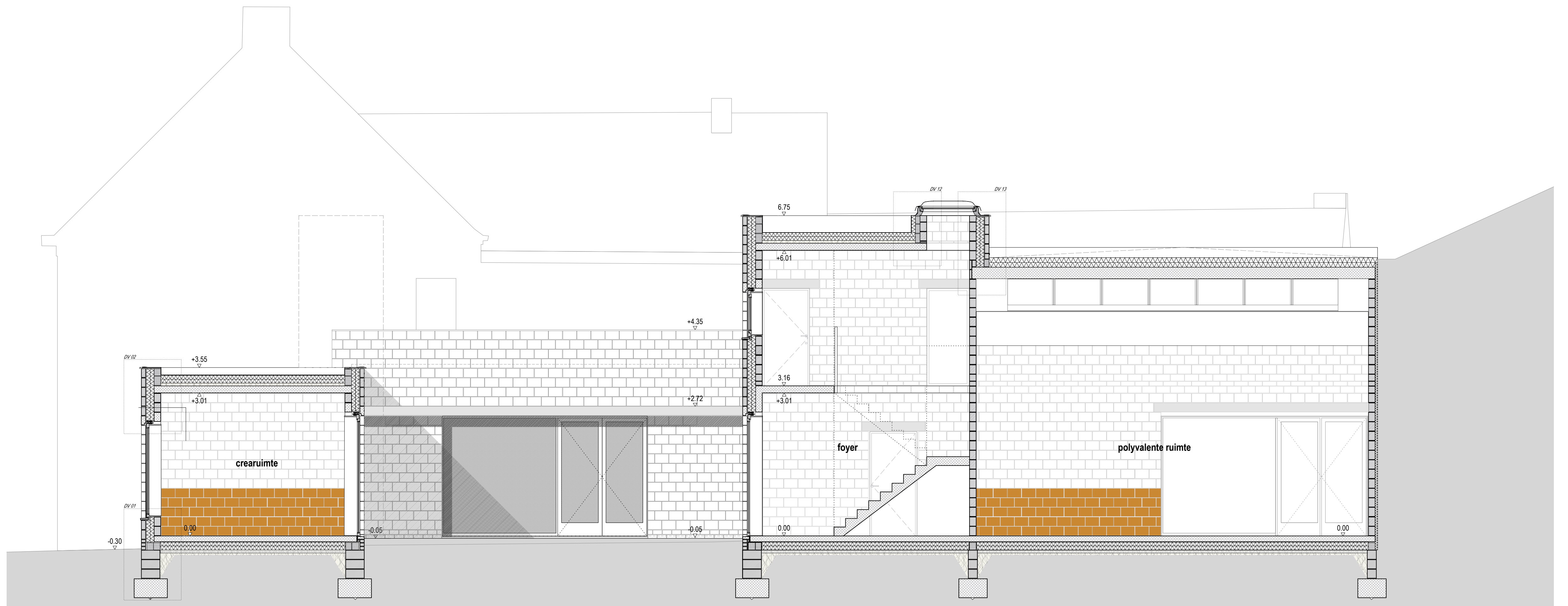
snede AA - 1/50
