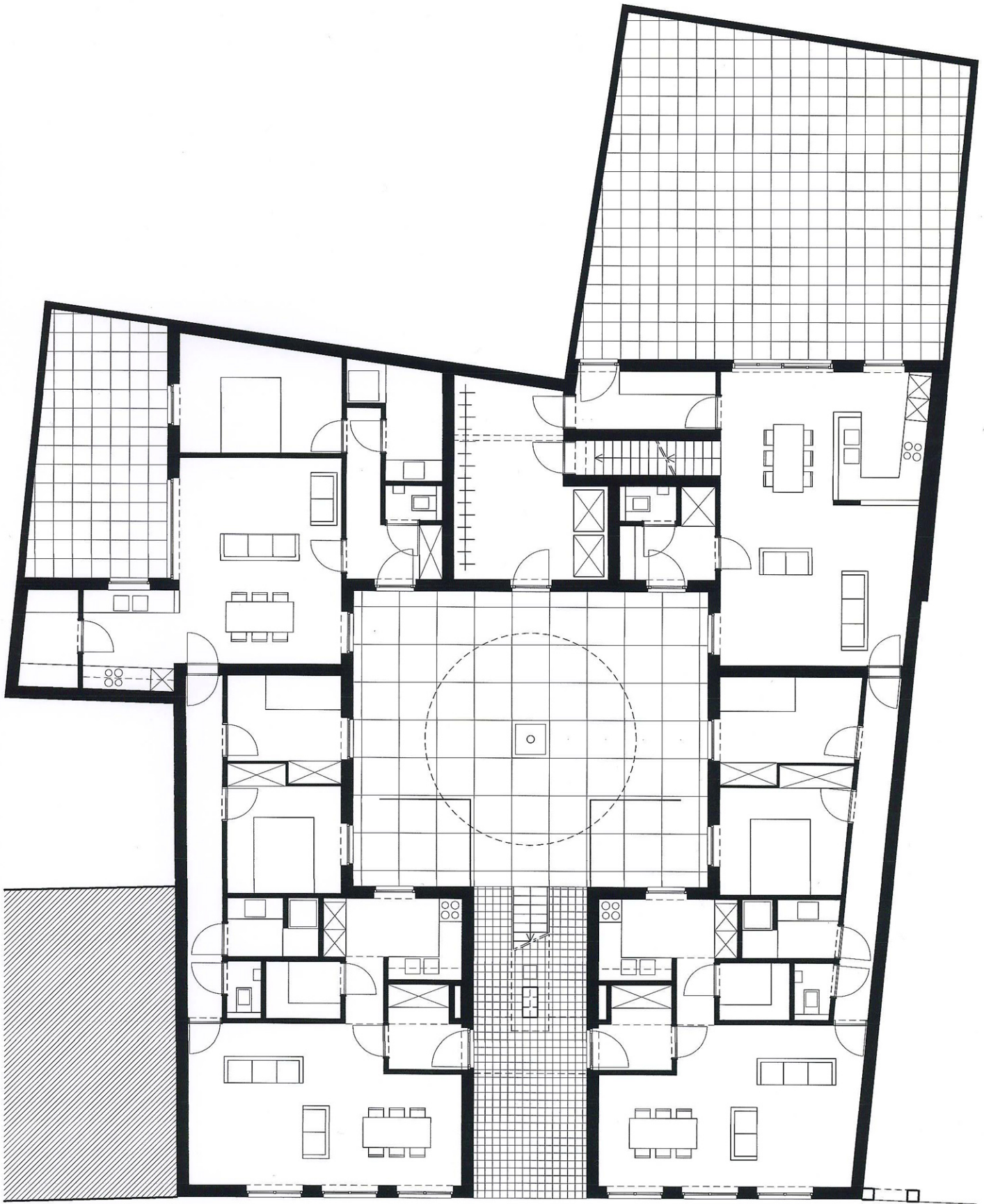
PLAN GELIJKVLOERS
