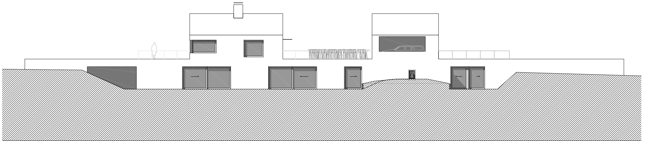
ZUIDGEVEL
