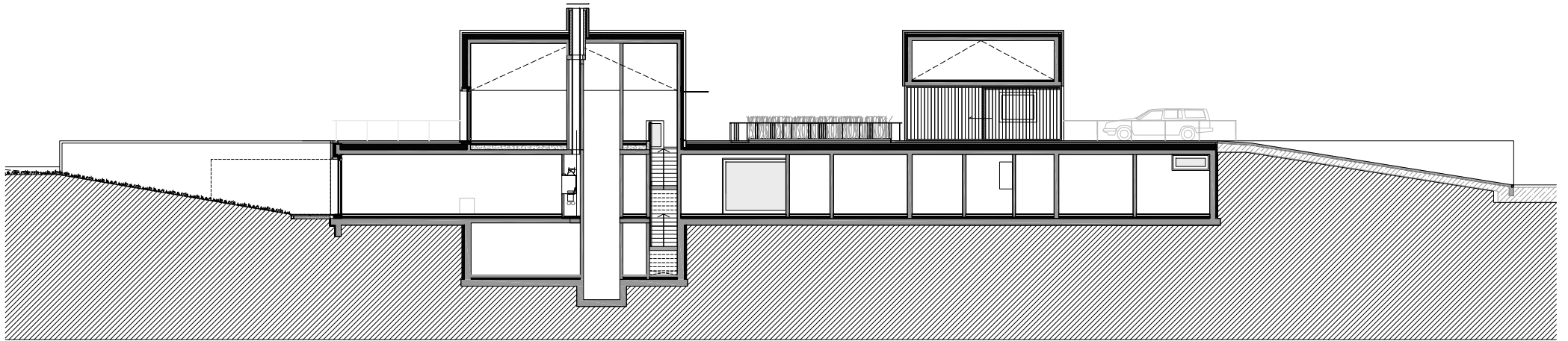
LANGSSNEDE
