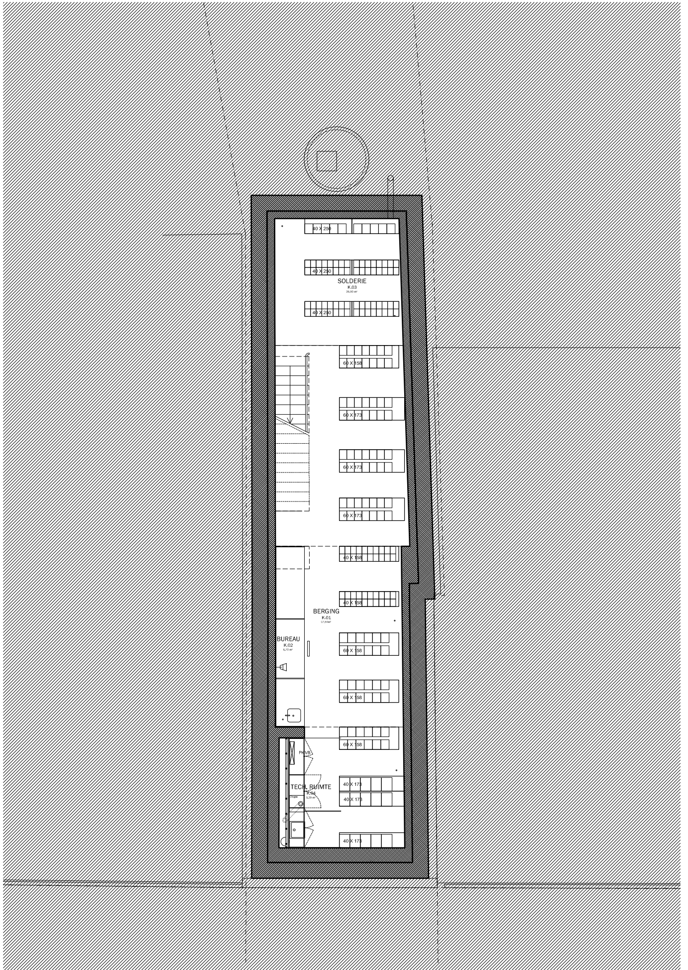
tekening 2 - verdieping -01 - 030 Kinderschoenen Deruyte - ONO architectuur
