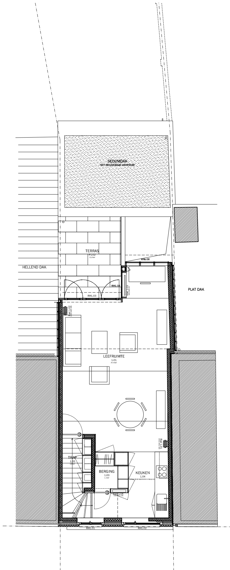
tekening 4 - verdieping 01 - 030 Kinderschoenen Deruyte - ONO architectuurr
