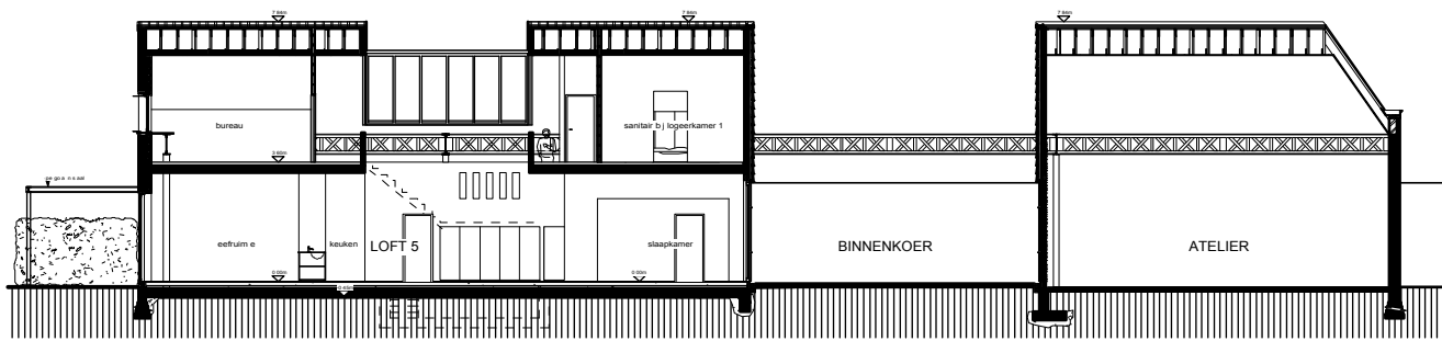
Doorsnede CC
