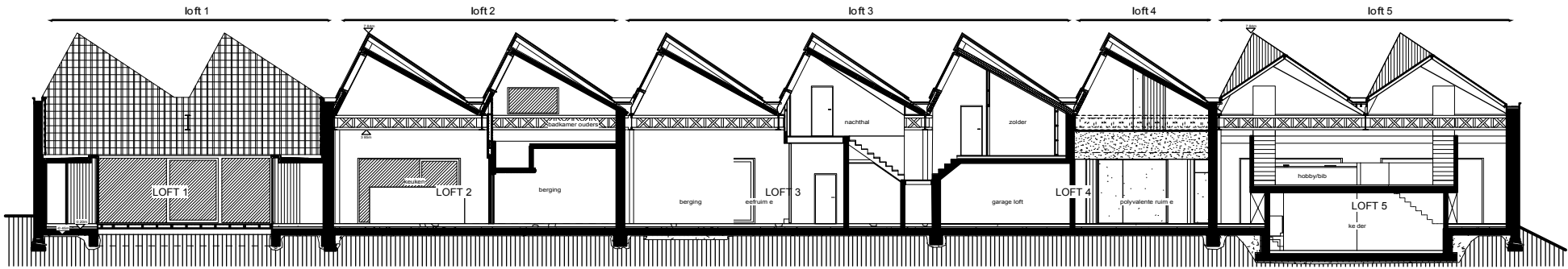
Doorsnede AA
