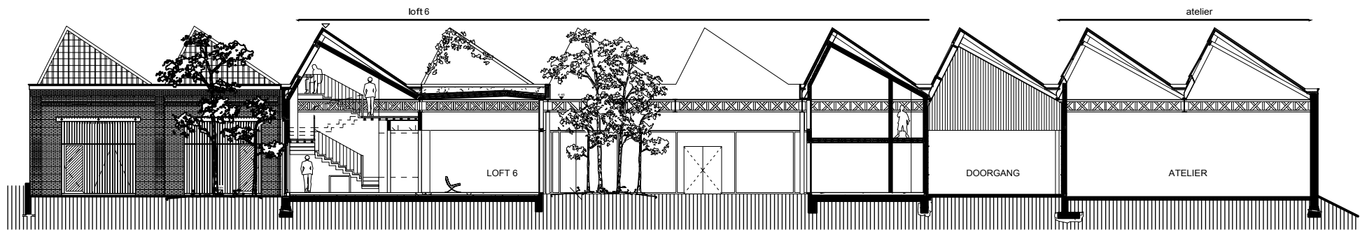
Doorsnede BB
