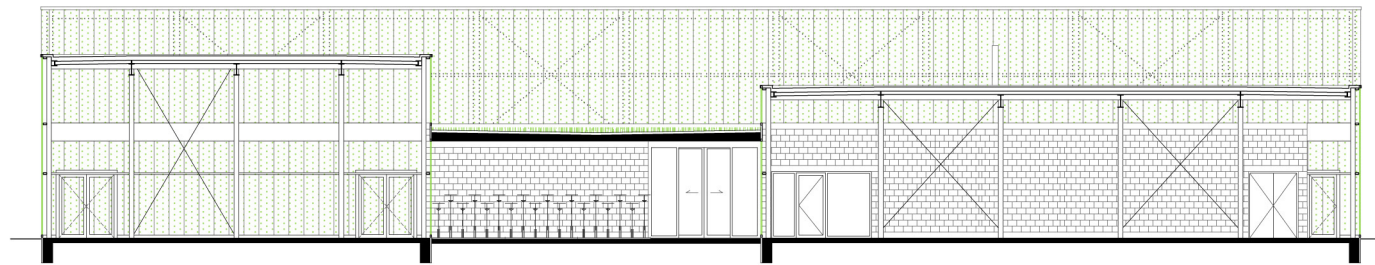
Doorsnede BB
