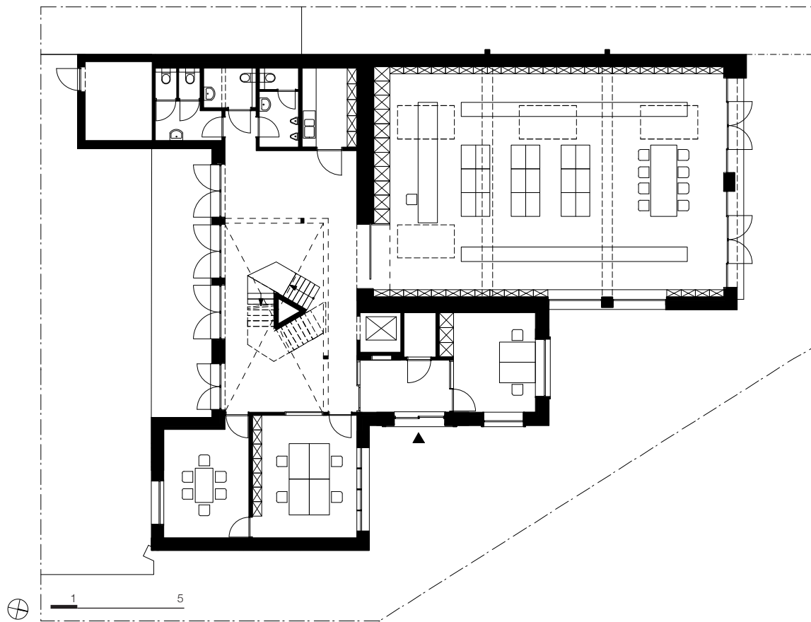
plan kazerne gelijkvloers nieuwe toestand
