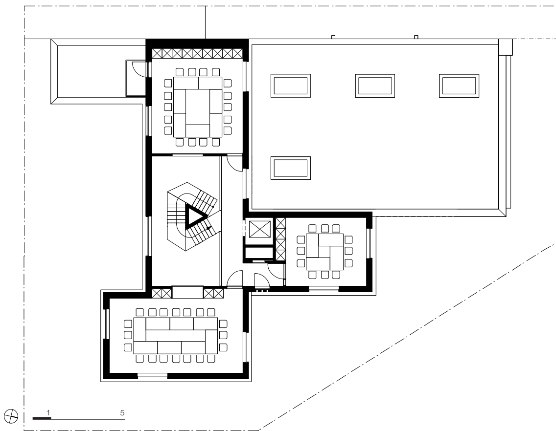
plan kazerne verdieping nieuwe toestand
