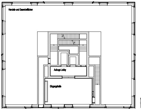
ERDGESCHOSS TURM 1
