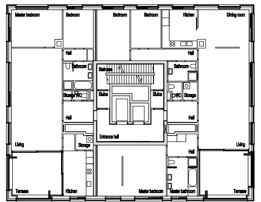
GESCHOSSTYP F
