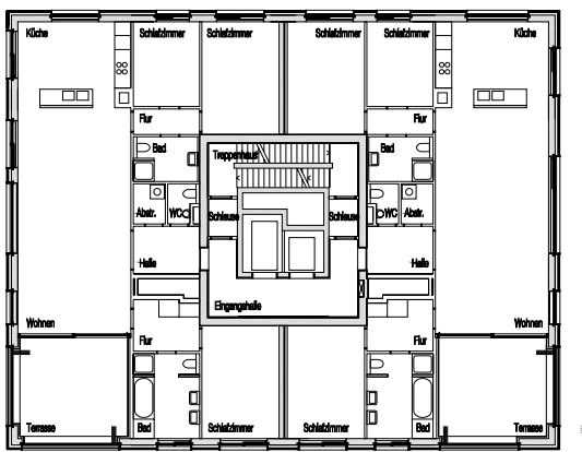
GESCHOSSTYP D
