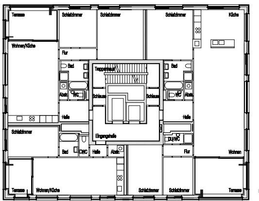
GESCHOSSTYP C
