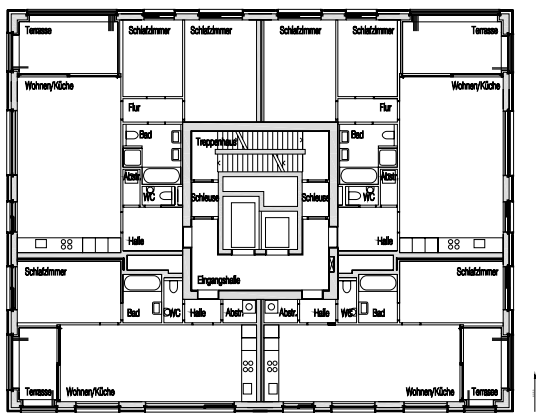
GESCHOSSTYP A
