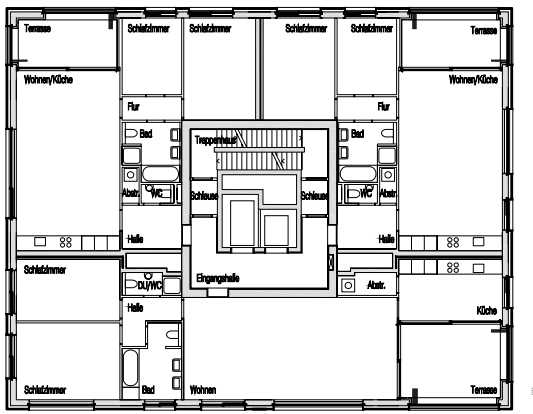
GESCHOSSTYP B
